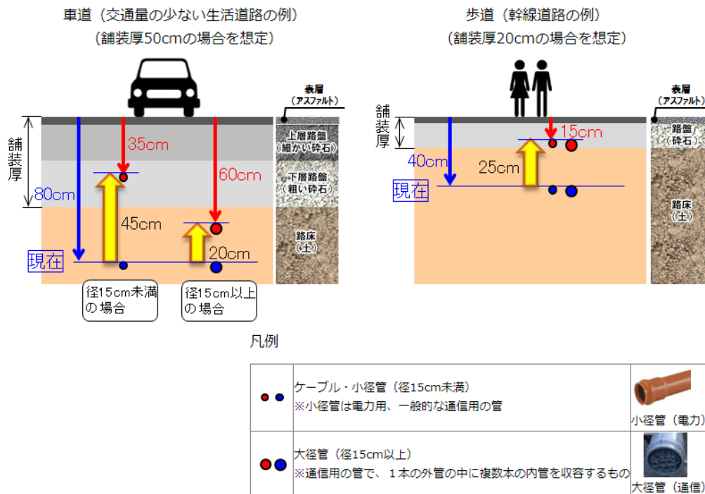
※舗装厚は、当該道路の交通状況、地盤状況に応じて設定される 図ー7 「電線等の埋設物に関する設置基準」の見直しイメージ図（出典：国土交通省HP）
